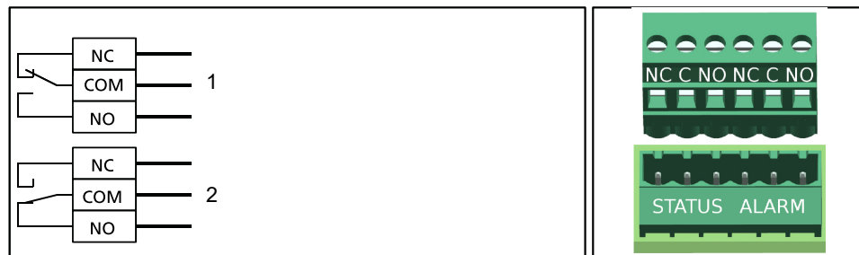
Рис. 11: Электрическая схема подключения, общий сигнал неисправности
