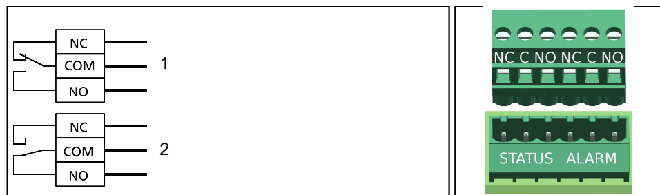
Рис. 10: Электрическая схема подключения, сообщение о режиме работы
