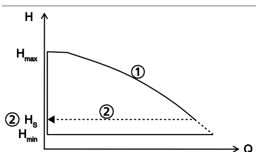
Рис. 20: Функция поддержания постоянного давления
