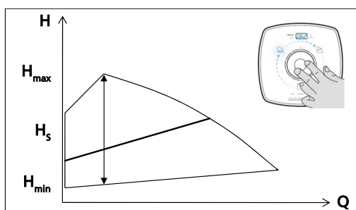
Рис. 23: Настройка режима пропорционального регулирования давления
