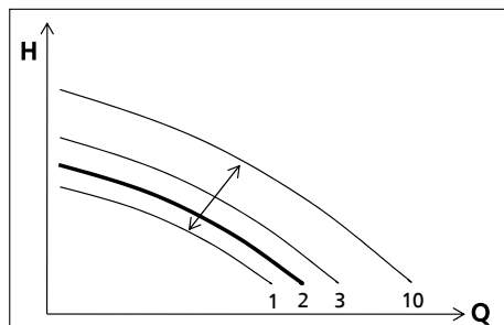
Рис. 26: Режим ручного регулирования, ступень частоты вращения 2
