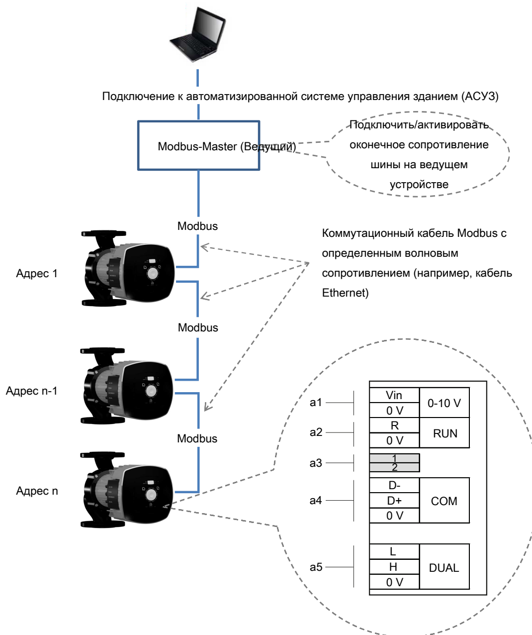
Рис. 14: Кабельное соединение насосных агрегатов через Modbus
