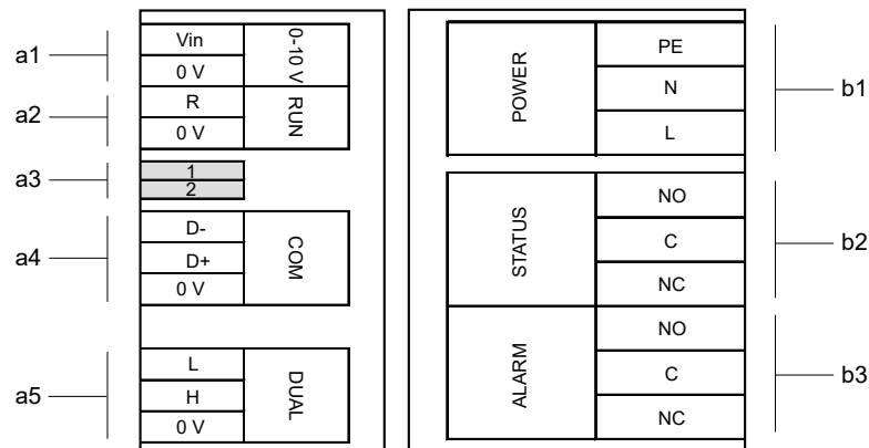
Рис. 31: Электрическая схема подключения
