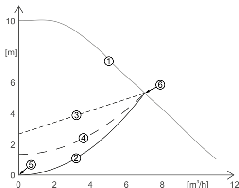
Рис. 24: Режим Есо и режим пропорционального регулирования давления на примере типоразмера 25-100
