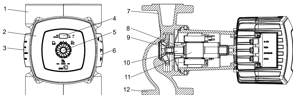
Рис. 5: Изображение насосного агрегата
