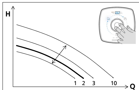
Рис. 27: Настройка режима ручного регулирования
