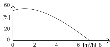
Рис. 25: Потенциал экономии в режиме Есо по сравнению с режимом пропорционального регулирования давления на примере типоразмера 25-100
