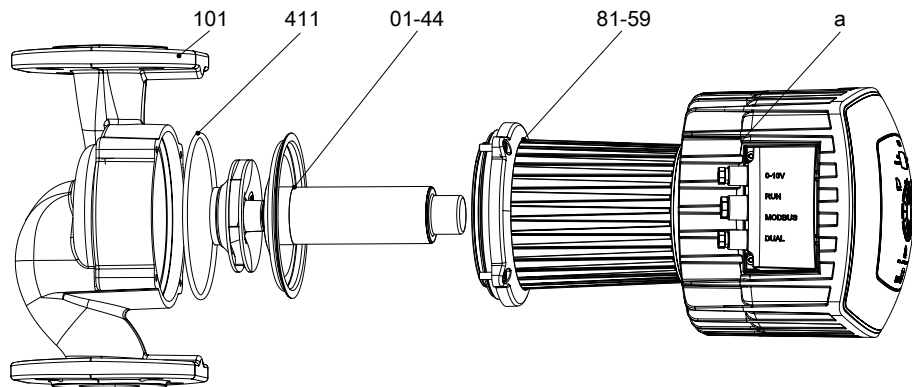
Рис. 30: Покомпонентный сборочный чертеж
