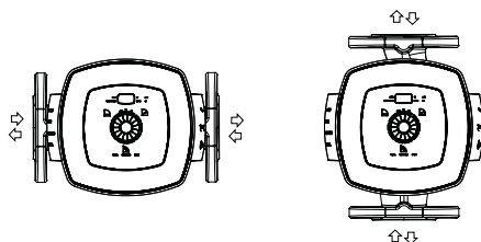
Рис. 7: Допустимые монтажные положения
