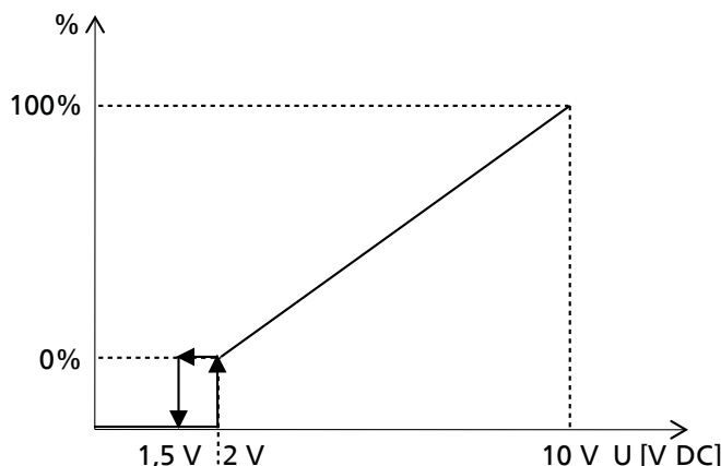
Рис. 28: Аналоговый сигнал 0 – 10 В для ввода заданного значения на насосном агрегате
