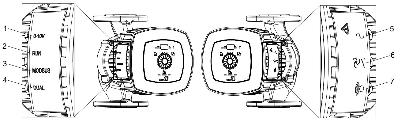
Рис. 8: Подключение электрических кабелей
