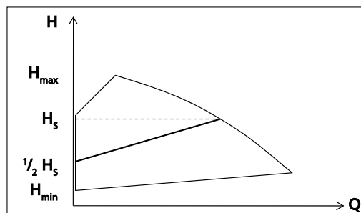
Рис. 22: Функция пропорционального регулирования давления
