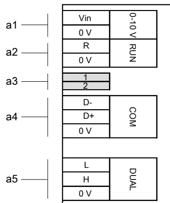
Рис. 17: Схема расположения клемм для двухнасосного режима работы
