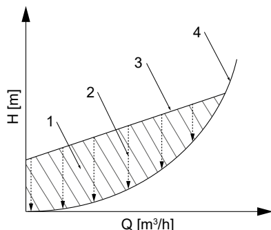
Рис. 29: Принцип динамического управления
