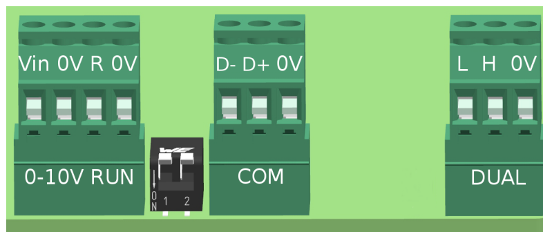
Рис. 16: Изображение клемм
